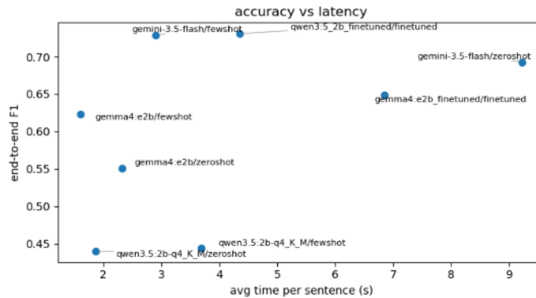
Slika 4.3. Odnos između prosečnog vremena izvršavanja po rečenici i end-to-end F1 mere za različite kombinacije modela i režima
