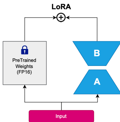
Slika 3.4. Princip rada LoRA metode [12]
