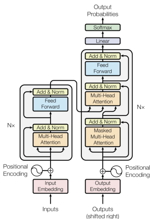
Slika 3.1. Transformer arhitektura [5]
