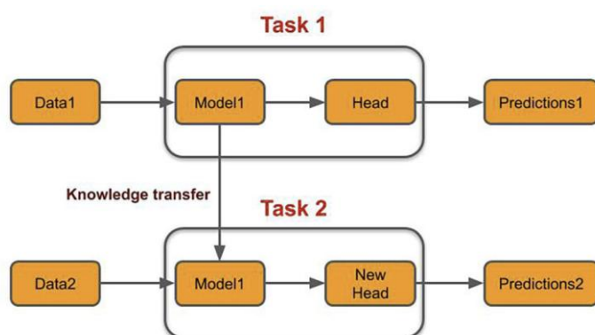
Slika 3.2. Preneseno učenje [8]
