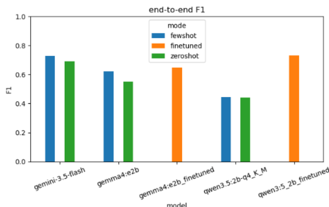
Slika 4.2. End-to-end F1 grafik po modelu/režimu
