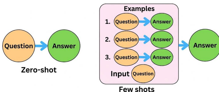
Slika 3.3. Razlika između zero-shot i few-shot pristupa
